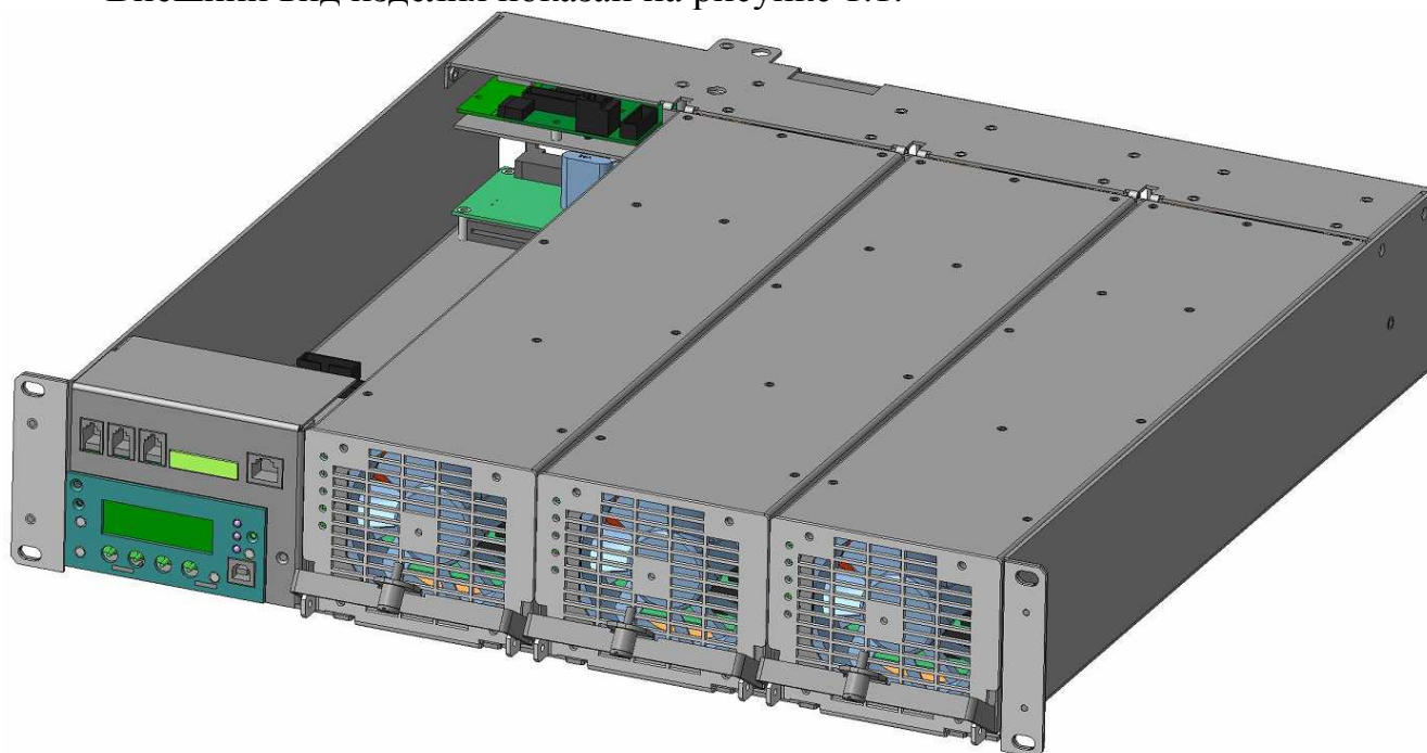
Рисунок 1.1 - Модульный каркас PS2000KM с инверторами PS48-60/2000К и контроллером Штиль PSC-200.03
